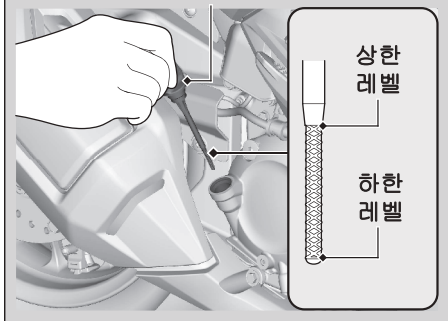
오일 주입구 캡/딥스틱
