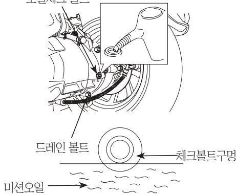
오일체크 볼트
