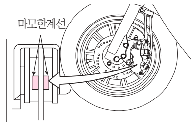
후론트 브레이크
