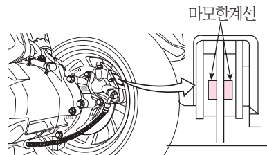
리어 브레이크
