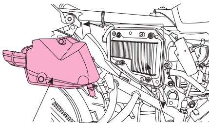
에어크리너 커버
