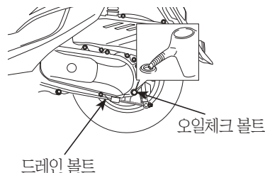
드레인 볼트
