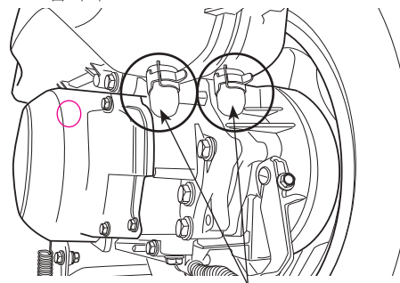
드레인 튜브
