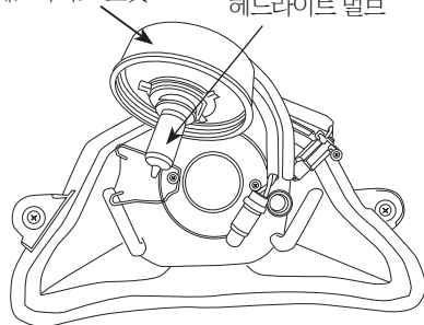
헤드라이트 소켓
