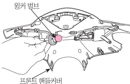
후론트 윙커 벌브규격
