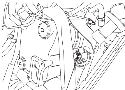
스파크 플러그
