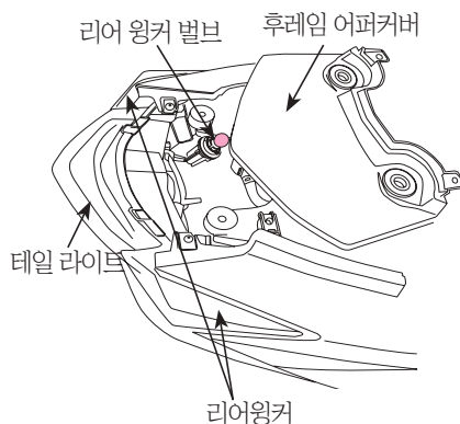
리어윙커 밸브규격
