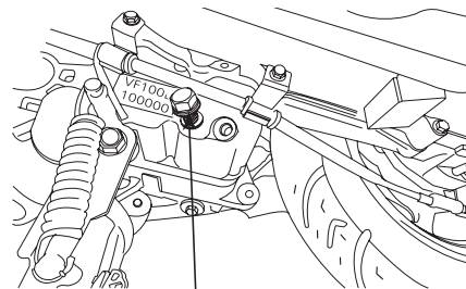
오일 드레인 볼트
