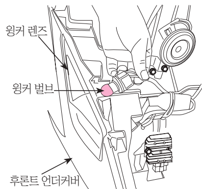
후론트 윙커 벨브규격
