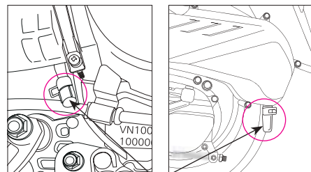
드레인 튜브
